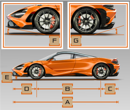
Dimensions - 765LT
