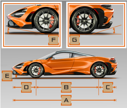
Dimensions - 765LT Coupe and Spider
