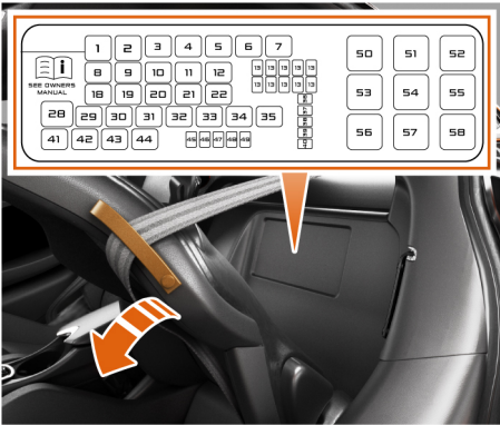
Cuadro de especificaciones de fusibles de la caja de fusibles principal
