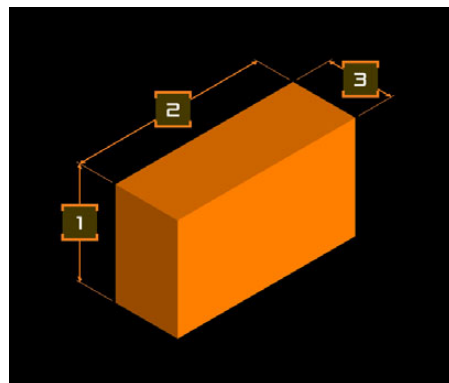
乘客座腳踏區置物網之物品最大體積 2 - 100 公釐高 (1) x 200 公釐寬 (2) x 70 公釐深 (3)。
