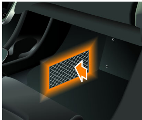
乘客座腳踏區置物網之物品最大體積 1 - 250 公釐高 (1) x 200 公釐寬 (2) x 20 公釐深 (3)。
